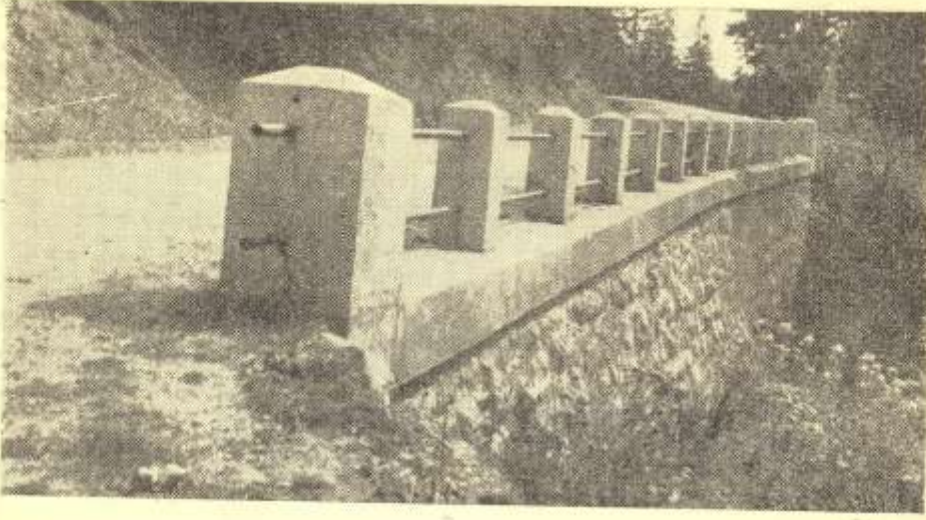
Çankırı - Kastamonu yolunda istinat duvarı
